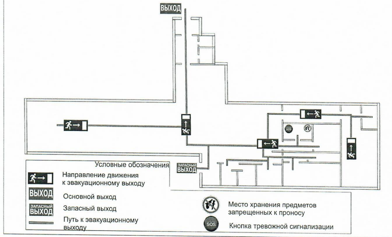
Схема расположения эвакуационных знаков и мест хранения предметов запрещенных к проносу «Стрелковый тир» с.п. Солнечный, ул. Зои Космодемьянской, 196
